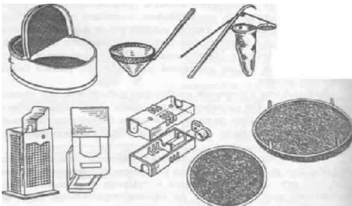
Рис. 37 - Инвентарь, используемый при размножении пчелиных семей и выводе маток: роевни разных видов (верхний ряд); маточные клеточки и колпачки для подсадки маток (нижний ряд).
