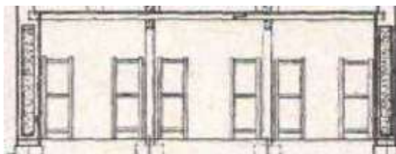
Рис. 49 - Поперечный разрез зимовника на 300 пчелиных семей
