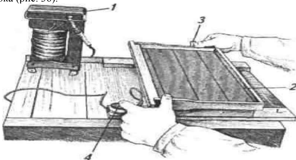
Рис. 36 - Электронаващивание рамок: 1 - пчеловодная проволока; 2 - вошина, размещённая на доске-лекало; 3 - выводные контакты источника электротока; 4 - электронаващиватель.
