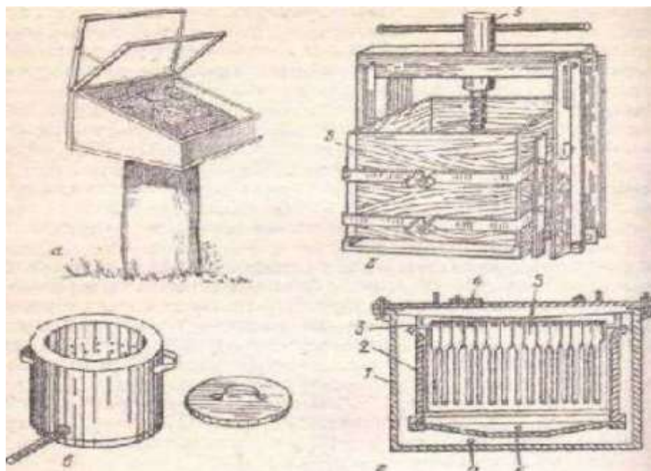
Рис. 43 - Инвентарь для переработки воскового сырья на пасеке: а - солнечная воскотопка; б - воскопресс; в - паровая воскотопка (для переработки воскосырья); г - паровая воскотопка для переработки сотовых рамок.
