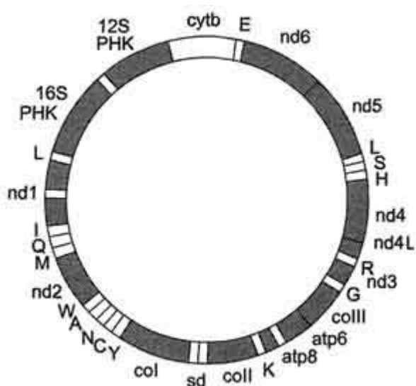
Рис. 14. Кольцевая молекула митохондриальной ДНК. Гены nd1-nd6 , nd4l кодируют субъединицы NADH-дегидрогеназного комплекса; ген coi-III - субъединицы цитохромоксидазы; ген cytb - цитохром Ь. Гены atp 8 и atp 6 кодируют субъединицы АТФ-синтазы (NADH-дегидрогеназный комплекс, цитохромоксидаза, цитохром b - белки, участвующие в энергетическом обмене). Остальные гены кодируют рибосомные (12S РНК и 16S РНК) и транспортные РНК соответствующих аминокислот, обозначенные латинскими буквами.
