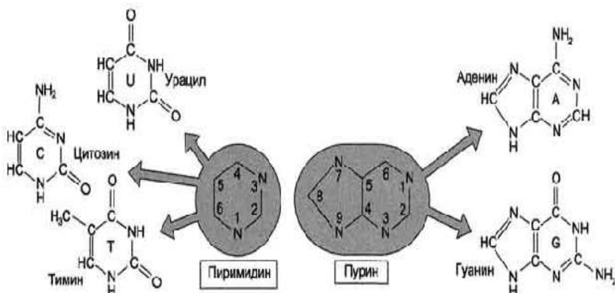
Рис. 7. Пуриновые и пиримидиновые основания.
