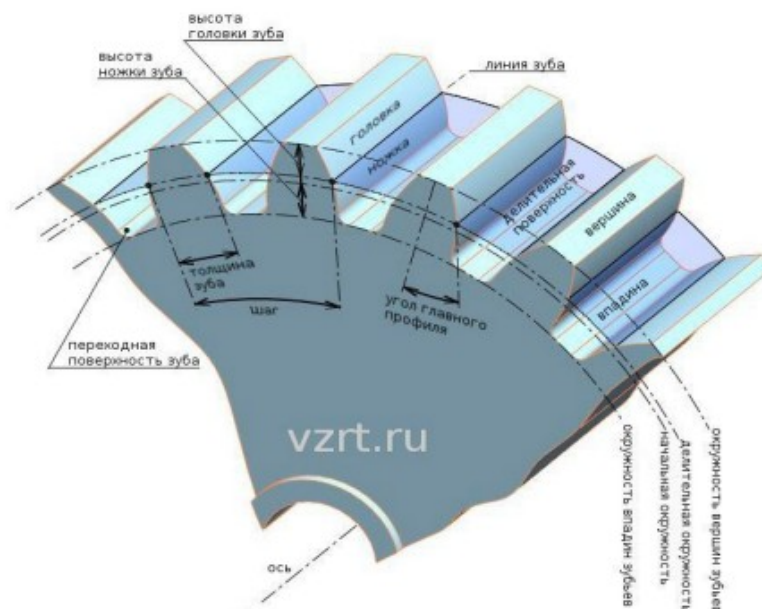
Рис. 1 Зубчатое колесо
