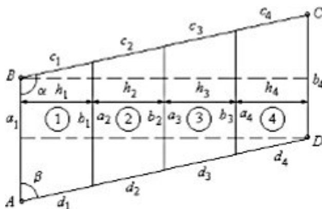
Рисунок 11 – Схема к проектированию участков равной площади линиями параллельными заданному направлению
