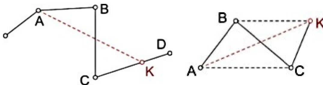
Рисунок 19 - Схемы к спряmlению границы путем графических построений
