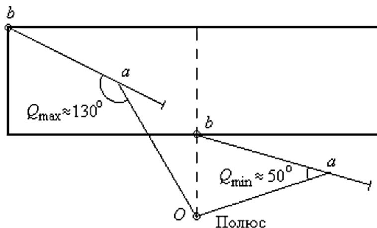
Рисунок 5 – Схема работы планиметром
