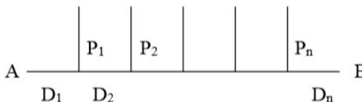
Рисунок 22 - Схема к перенесению в натуру методом промеров
