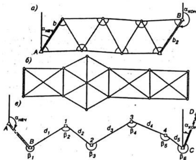
Рисунок 3 - Методы планового обоснования геодезических сетей:
