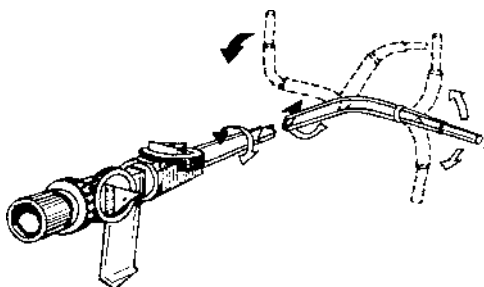
Рис. 3.5 Схема управления изгибом дистального конца в волоконном эндоскопе
